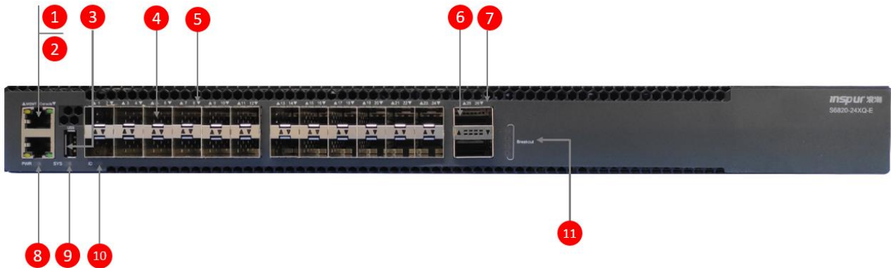
图 1-1 S6820-24XQ-E 前面板示意图
