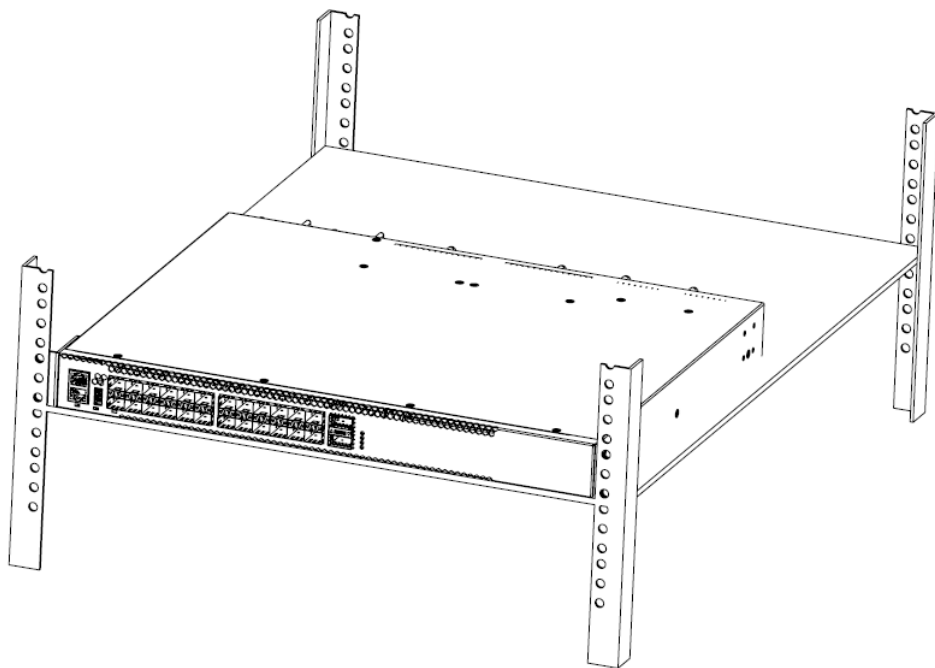
图 2-3 交换机安装至机架（带托盘）示意图
